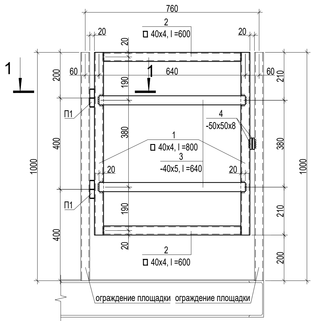
Калитка ограждения К1
