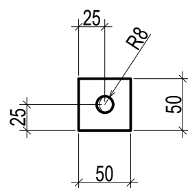
Деталь поз. 4
